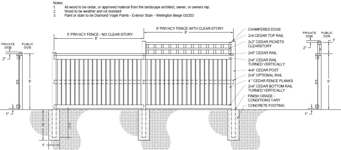
2 WOOD PRIVACY FENCE Scale: N.T.S.
