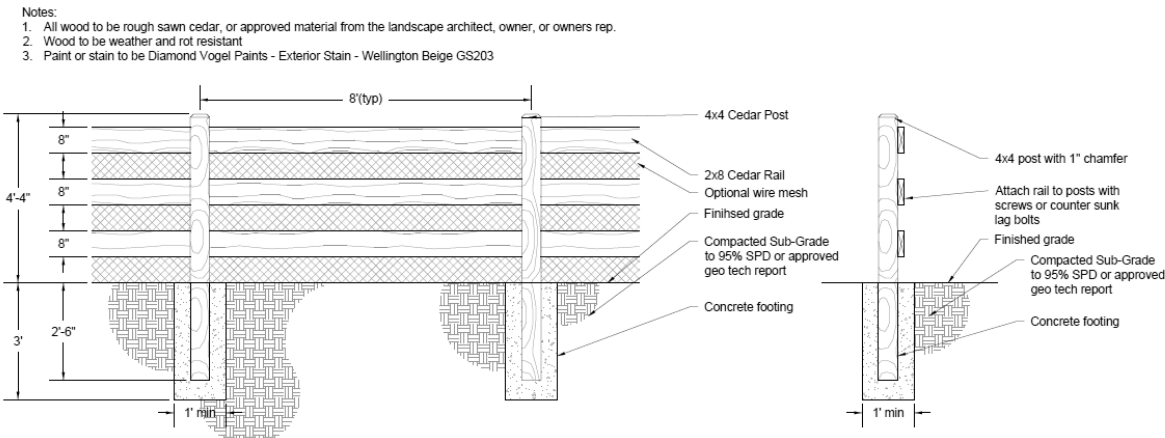
1 OPEN RAIL FENCE Scale: N.T.S.
